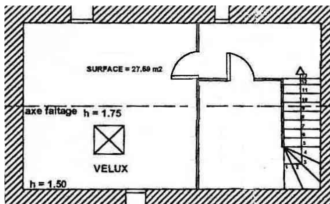
Tweede verdieping, Zweiten Stock, Second Floor, deuxième étage, 40 m 2
