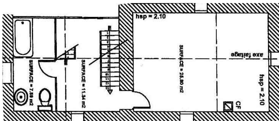
Erste verdieping, Ersten Stock, First floor, Premier étage, 45 m 2
