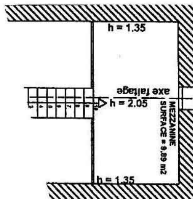
Tweede verdieping, Zweiten Stock, Second Floor, deuxième étage, 10 & 19 m 2
